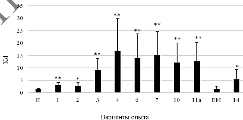
Рисунок 3 – Коэффициент распределения ^{137}\text{Cs} в торфяной почве
