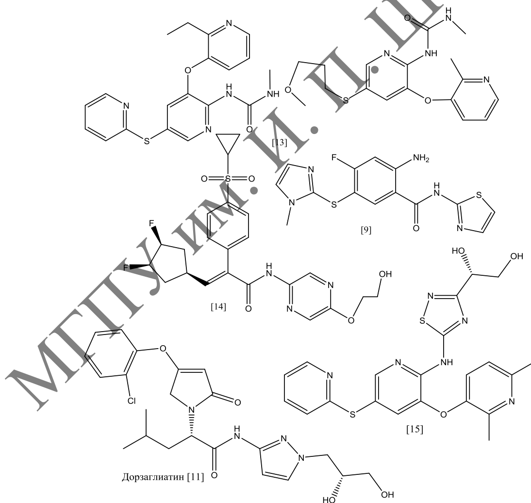
Рисунок 1 – Формулы потенциальных активаторов глюкокиназы (в скобках указаны ссылки на публикации)
